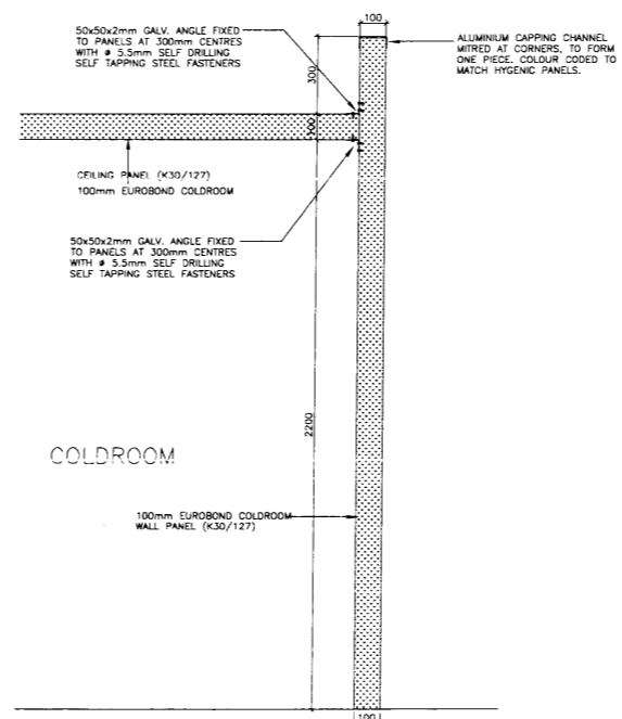
SECTION DD Scale 1:10
